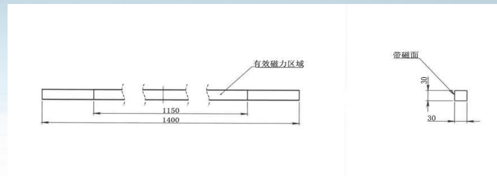
Magnetic rod
